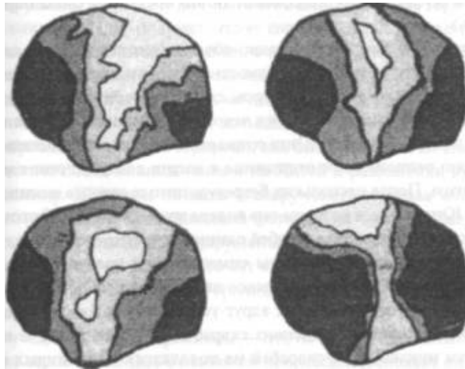
Рис. 10. Паттерны мозговых волн в случае четырех поединдивидуумов пациента, страдающего от множественного разделения личности. Использует ли мозг голографический принцип для хранения огромного количества информации, необходимой для размещения десятков или даже сотен личностей в одном теле? (Авторская копия с оригинальной работы Беннета Брауна в «American Journal of Clinical Hypnosis».)
