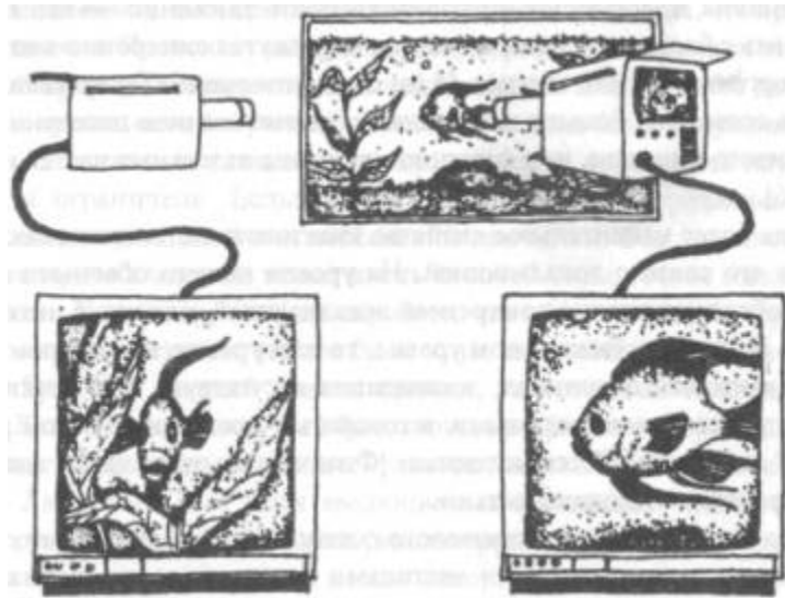
Рис. 8. Бом считает, что элементарные частицы связаны также, как изображения одной рыбы в двух гранях аквариума. Хотя частицы, наподобие электронов, кажутся отделенными друг от друга, на более глубоком уровне реальности – реальности аквариума – они являются лишь двумя аспектами глубокого космического единства.
