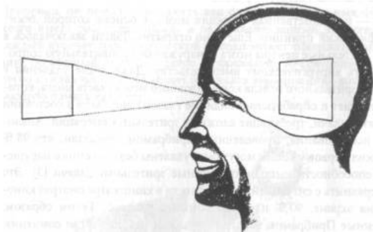
Рис. 5. Исследователи, занимающиеся теорией зрения, ранее считали, что существует взаимно-однозначное соответствие между видимым образом и тем, как он представлен в мозгу Прибрам обнаружил, что это не так
