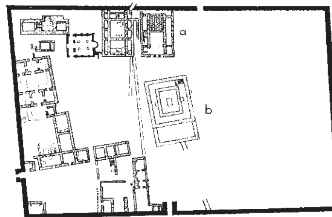
Plánek vnitřního hradu s pohanskou svatyní v Plisce (b) a plánek jiné pohanské svatyně pod palácovým kostelem (c, viz obr. na str. 168); vyznačen je též obytný dvorec (a)
