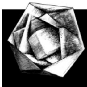
Obr. 22: Geometrický model atomového jádra Dr. Roberta Moona
