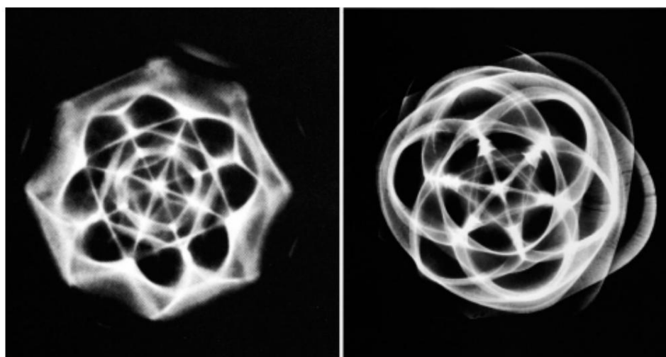
Obr. 21 : Ilustrace geometrie ve vibrující tekutině od Dr. Hanse Jennyho. Částice písku tvoří dva různé složité tvary, jak se mění frekvence zvuku.
