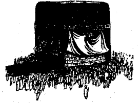
Kaaba.
