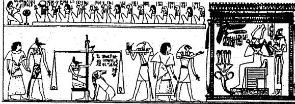
Uctívání Ustra.
