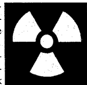
Značka radioaktivity.
