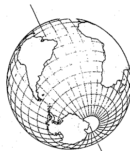
Precese.
